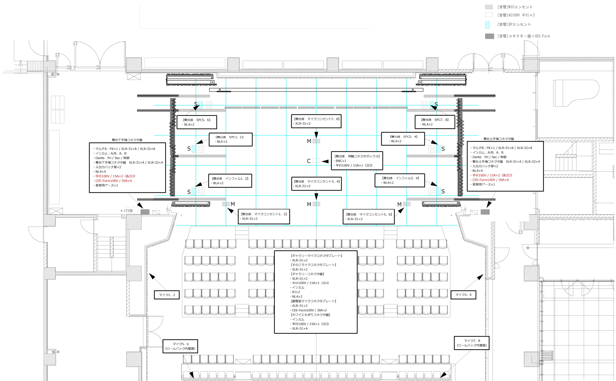
邑楽町中央公民館 ホール 音響コネクター盤配置図
